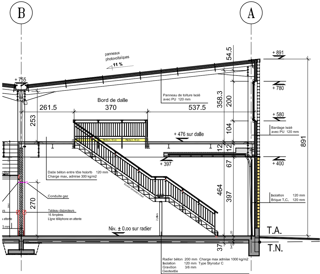
COUPE A-A
