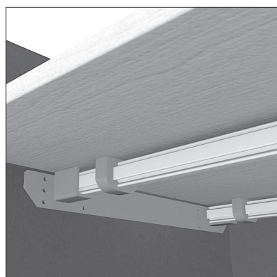
Plateau réglable en hauteur 3 hauteurs possibles : 720, 740 ou 760 mm
